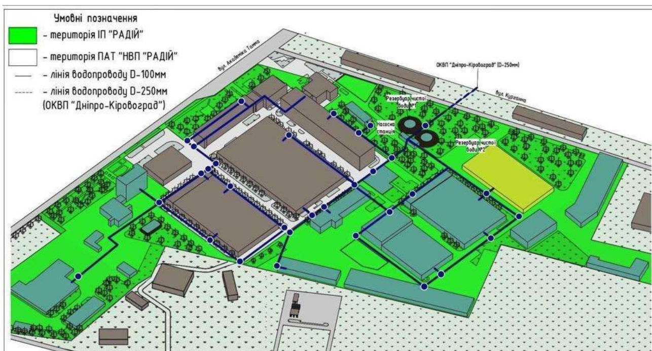
Мал. 5. Схема розташування мереж і об'єктів системи водопостачання
