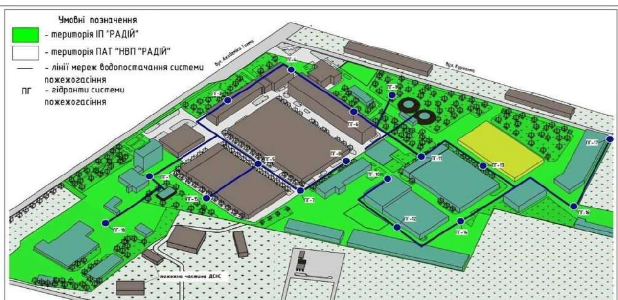
Мал.8 Схема розташування мереж та об'єктів системи пожежогасіння
